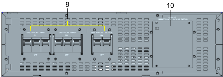
前视图(取下塑胶面板)
