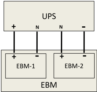
单一外部电池组（EBM）
