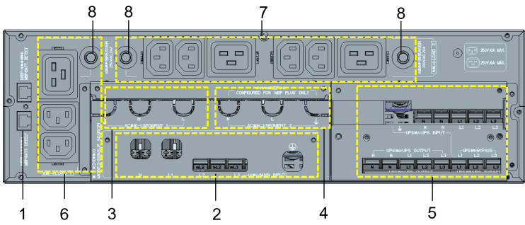
后视图
