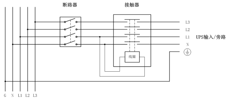
三相系统示意图
