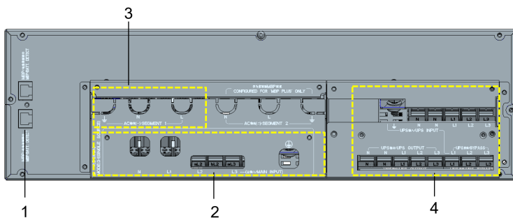
后视图
