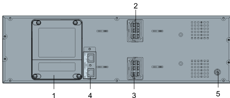
后视图
