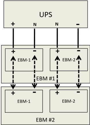
扩展外部电池组（EBM）
